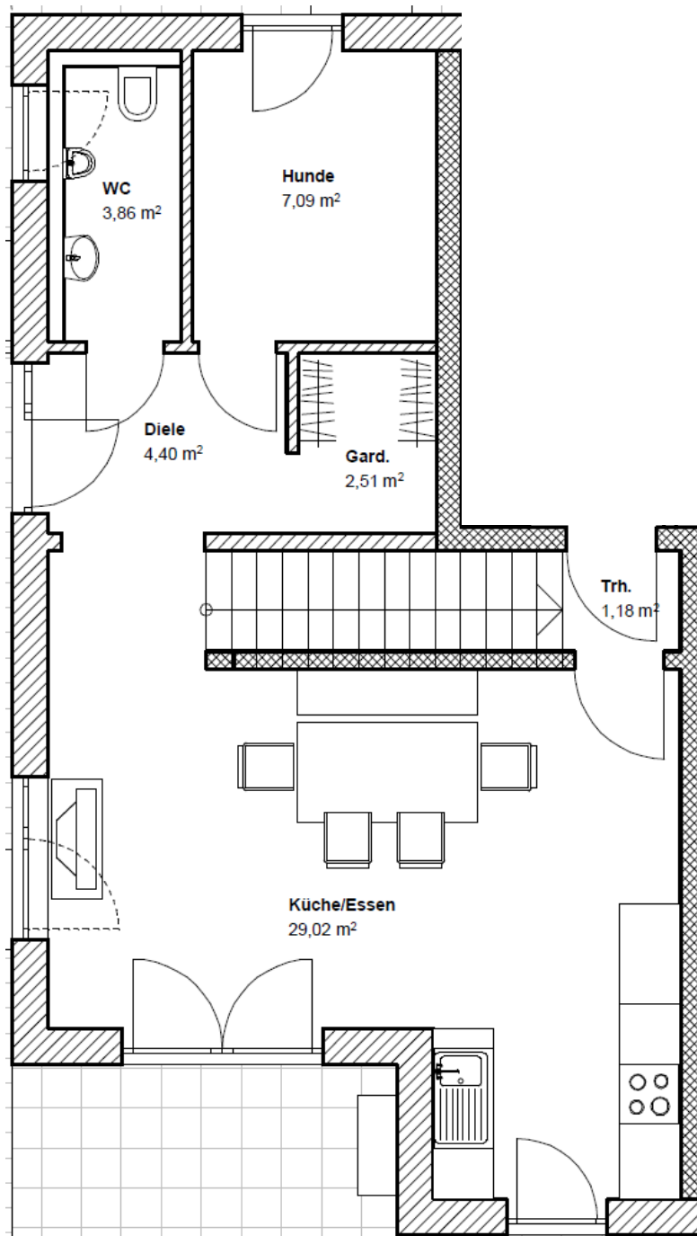
ERDGESCHOSS
