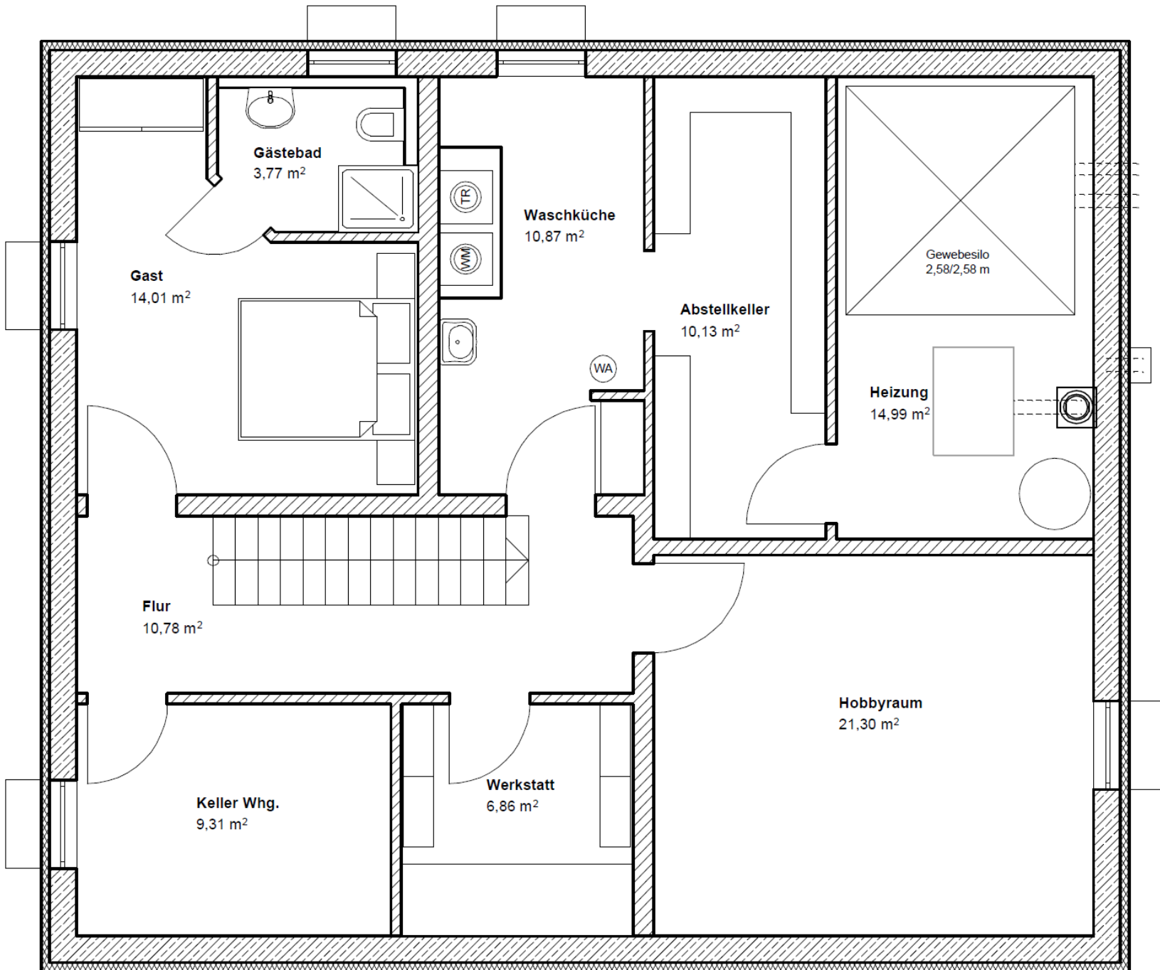
KELLERGESCHOSS
